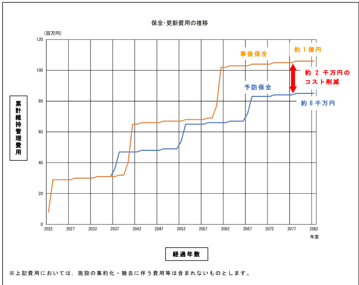
図6 保全・更新費用のシミュレーション
