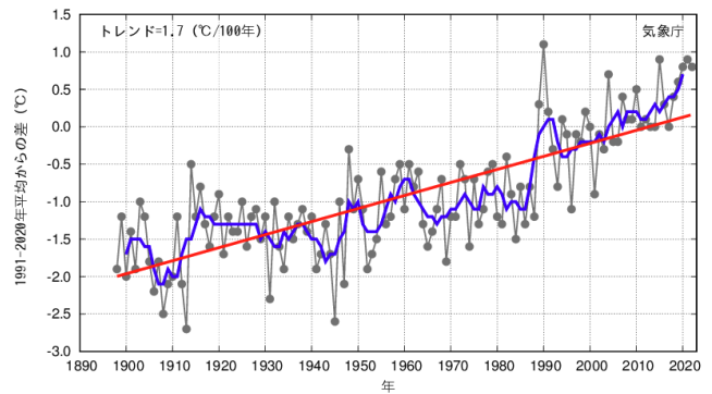
図2-2 函館の年平均気温偏差(1898~2022年)
