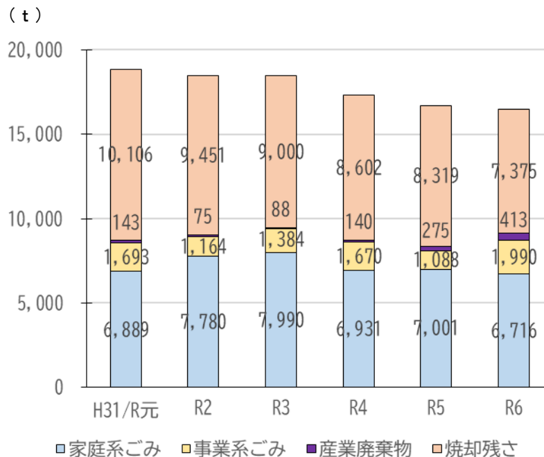
図 3.13 埋立処分量の推移（七五郎沢廃棄物最終処分場）
