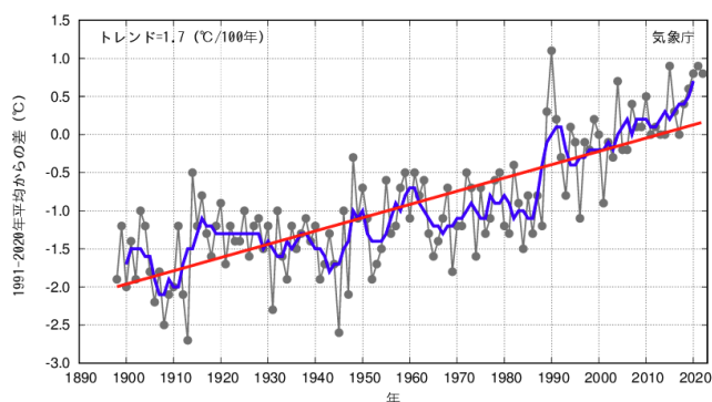
図2-2 函館の年平均気温偏差(1898~2022年)
