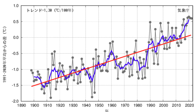
図2-1 日本の年平均気温偏差(1898~2022年)
