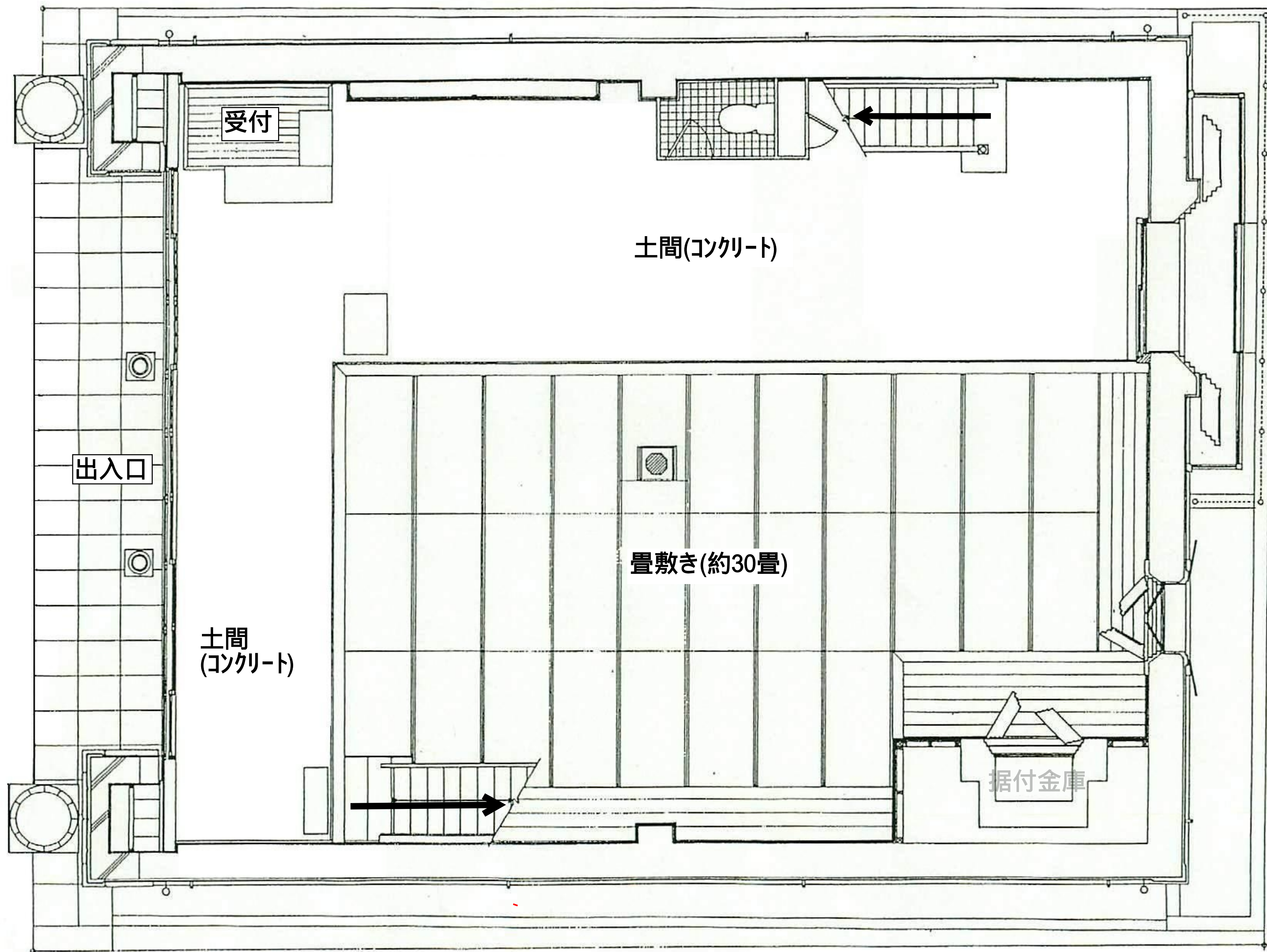
市立函館博物館郷土資料館(旧金森洋物店) 平面図(1階)
