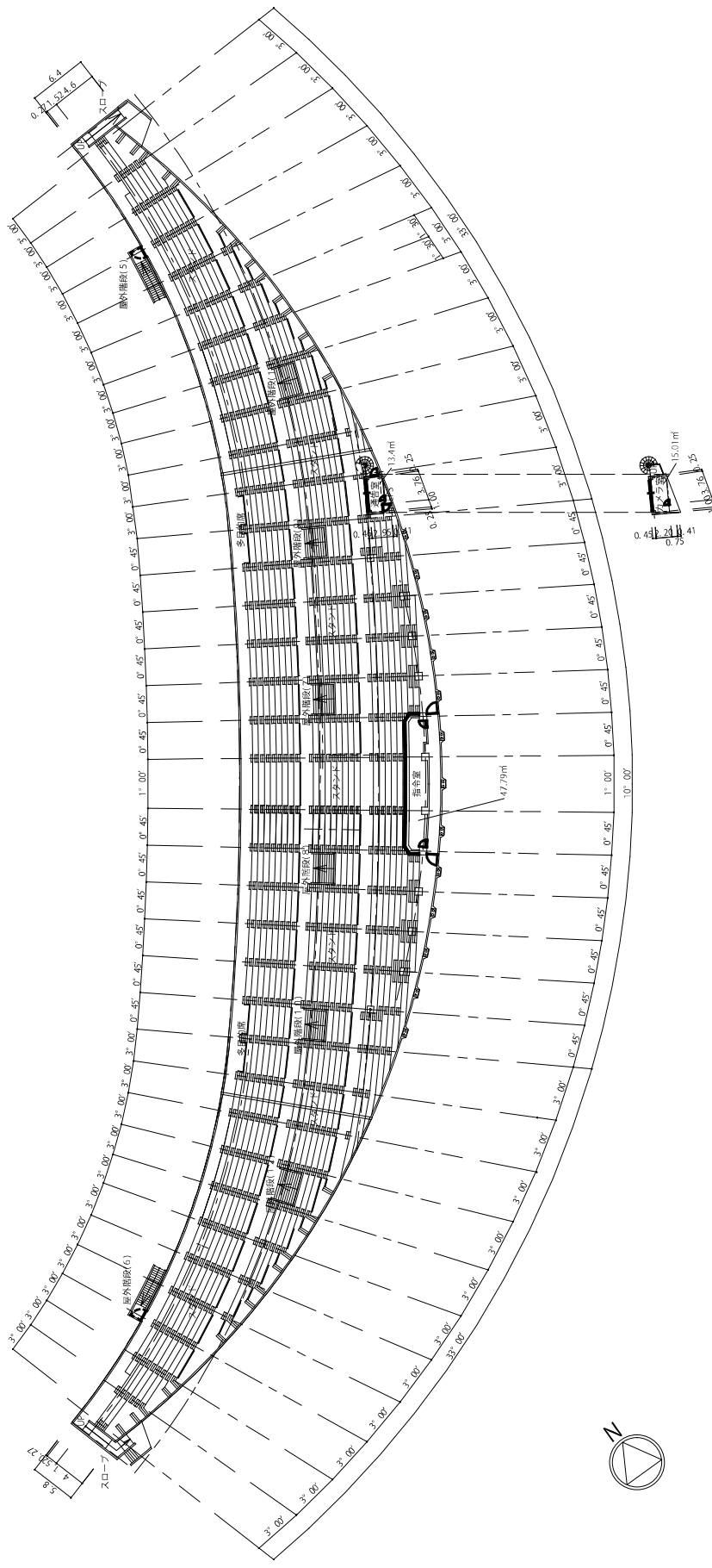
カメラ室階 S=1/600
