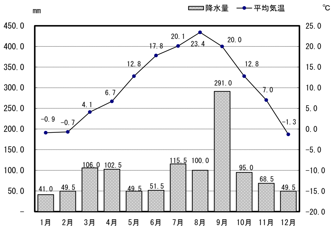
平均気温および降水量 (令和2年(2020年))
