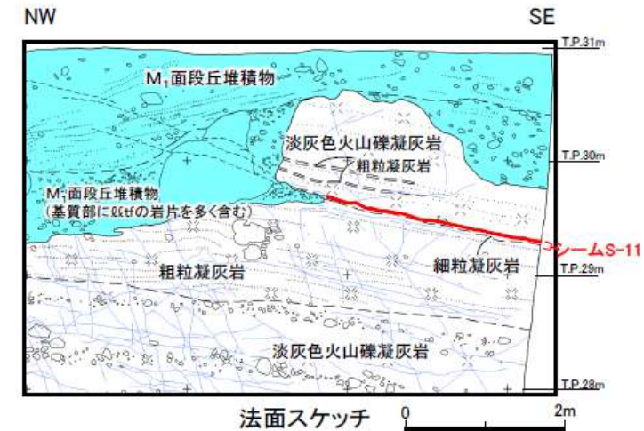
法面スケッチ
