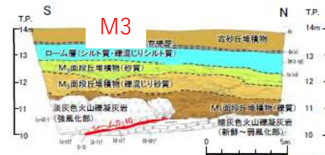
Ts-3トレンチ8m西側面: 変状が認められる (比高約14cm〔段丘堆積物中の層理面の段差〕) (補足説明資料P.4-40参照)
