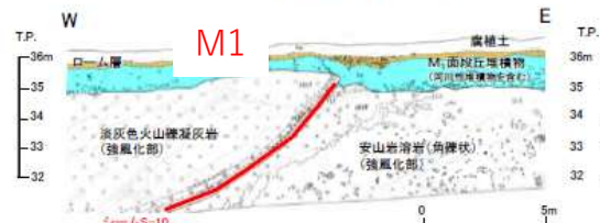
Ts-13法面北側面: 変状が認められる (比高約30cm*〔段丘堆積物上面の層理面の段差〕) (補足説明資料P.4-48参照)
