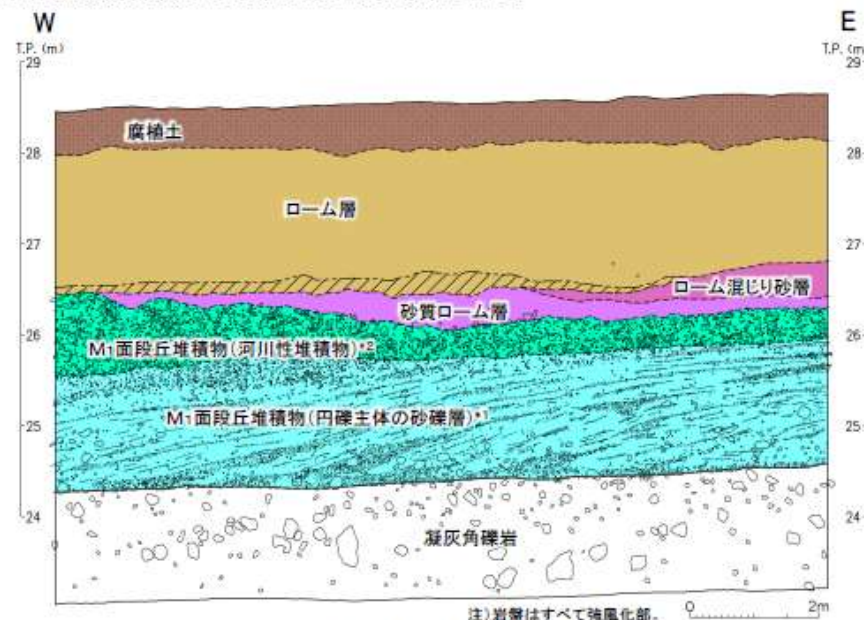
図2.3 法面④詳細スケッチ
