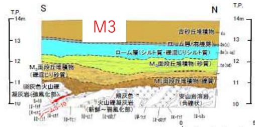
Ts-3トレンチ17m西側面: 変状が認められる (比高約9cm〔段丘堆積物中の層理面の段差〕) (補足説明資料P.4-41参照)
