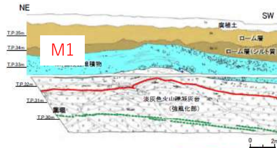
Ts-8トレンチ南側法面: 変状が認められる (比高約85cm[段丘堆積物の上に凸の形状]) (補足説明資料P.4-23参照)
