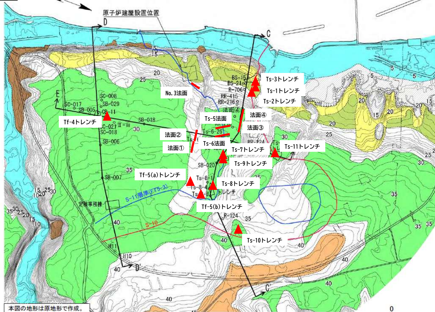
敷地の段丘面区分図に、S-10・S-11が第四系基底面等に現れる位置とトレンチや法面等の位置を重ねた図
