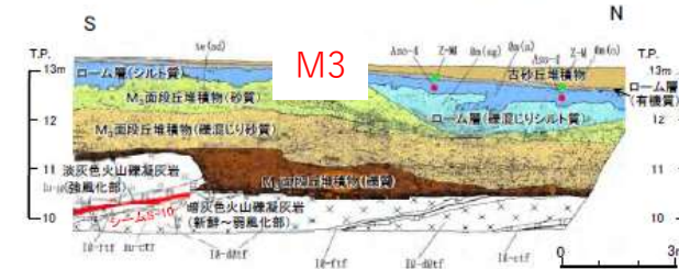
Ts-3トレンチ西側面: 変状が認められる (比高約25cm〔段丘堆積物中の層理面の段差〕) (補足説明資料P.4-35参照)
