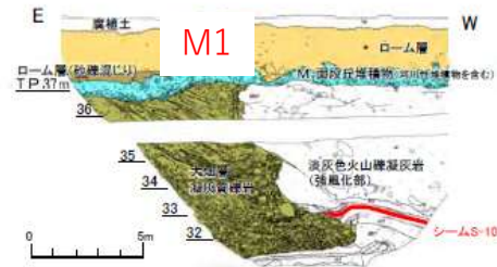
Ts-10トレンチ南側面: 変状が認められる (比高約65cm*〔段丘堆積物上面の層理面の段差〕) (補足説明資料P.4-46参照)
