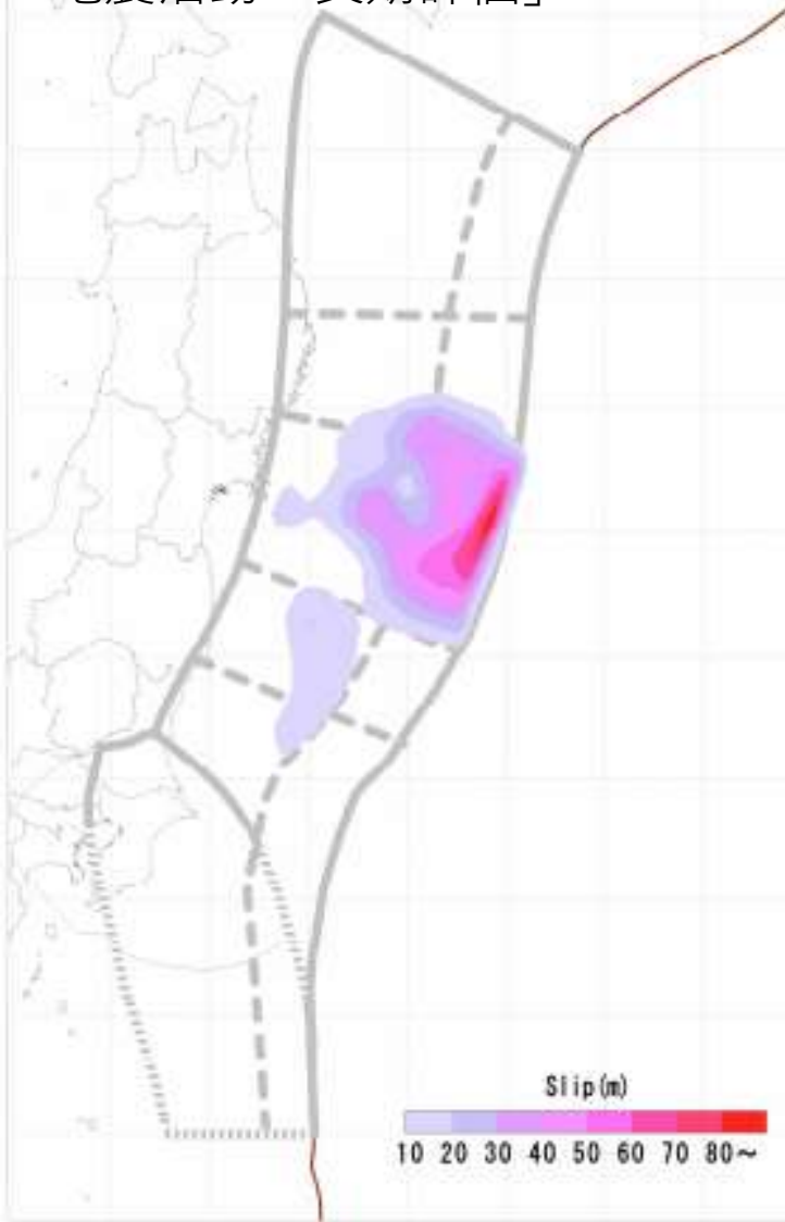
図4 東北地方太平洋沖地震の地震時のすべり量の分布 Iinuma et al. (2016) をもとに作成
