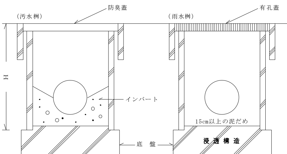
図-10 枡構造図
